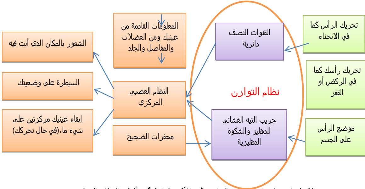
الشكل ( ١١ ) تواجد قنوات التوازن في الأذن الداخلية وتأليف النظام الدهليزي
